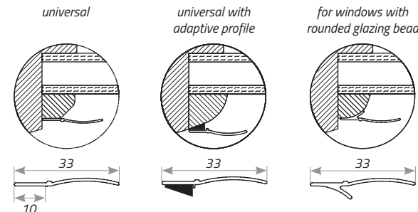
Fig.4 Side guide options
