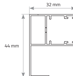
Bild 3 Führungs-Schiene mit Versetzprofil
