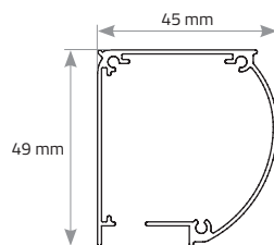
Bild 1 Kassetten Abschnitt
