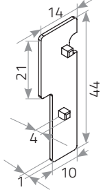
Mini Distanzplatte für Jalousie Venus
